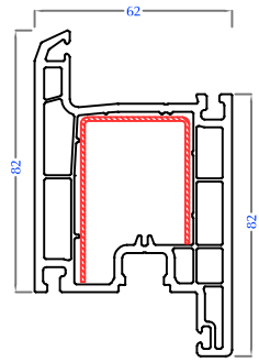
Door Sash - Inward Open PC62-US-04
