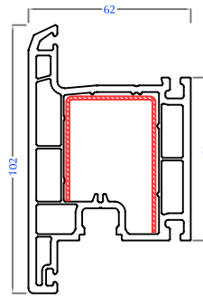
Door Sash - Outward Open PC62-US-03
