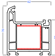
Door Frame PC62-UF-02
